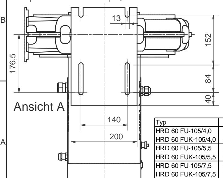
Ansicht A
