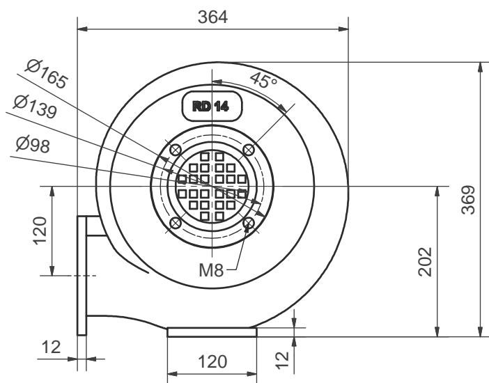
Ansicht A
